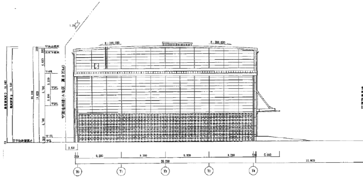
東立面図
